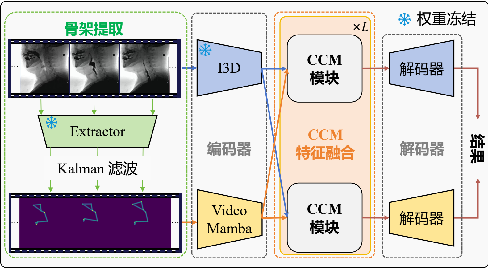
(a) SG-Mamba框架示意图
