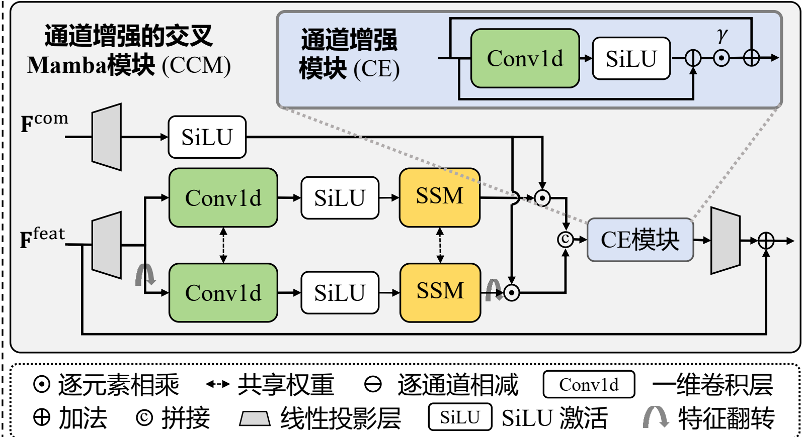
(b) CCM 模块示意图
